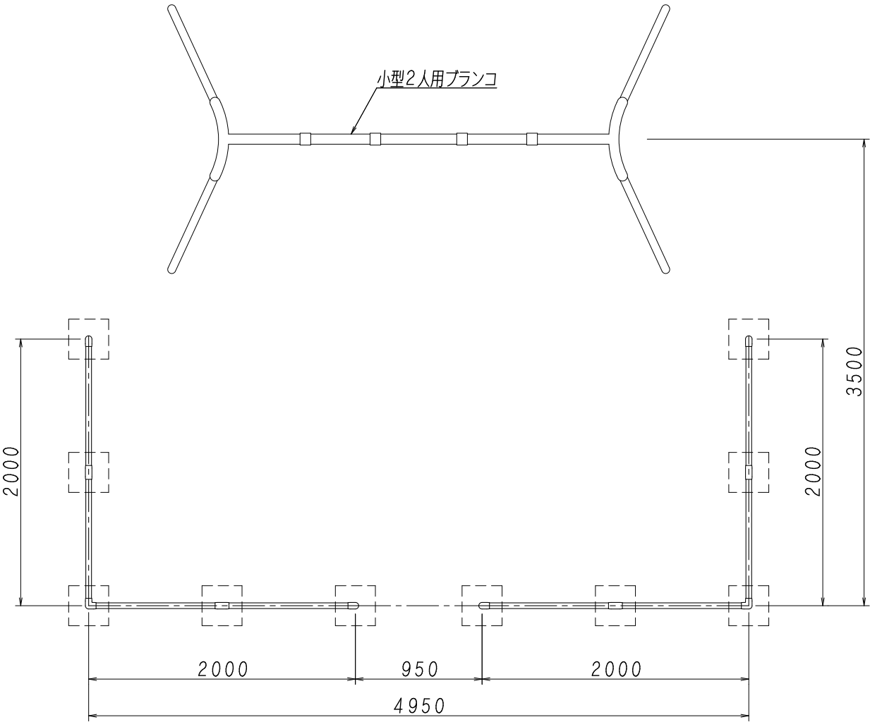
設置 平面図
