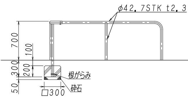
正面図
