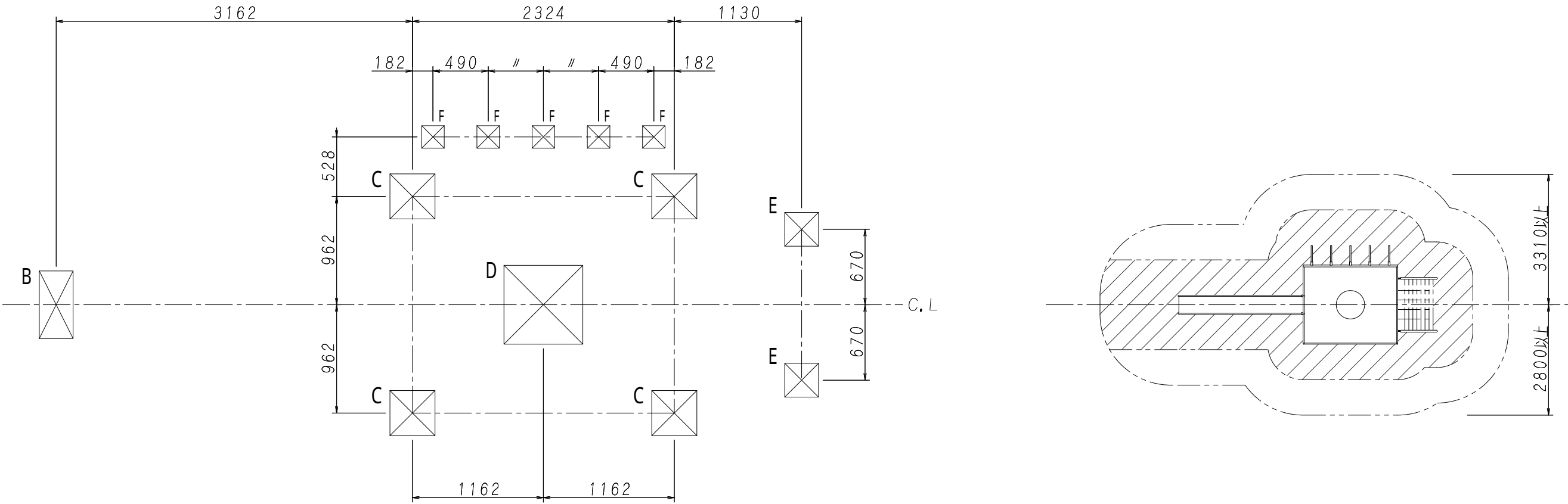
基礎平面図 S = 1 / 4 0
