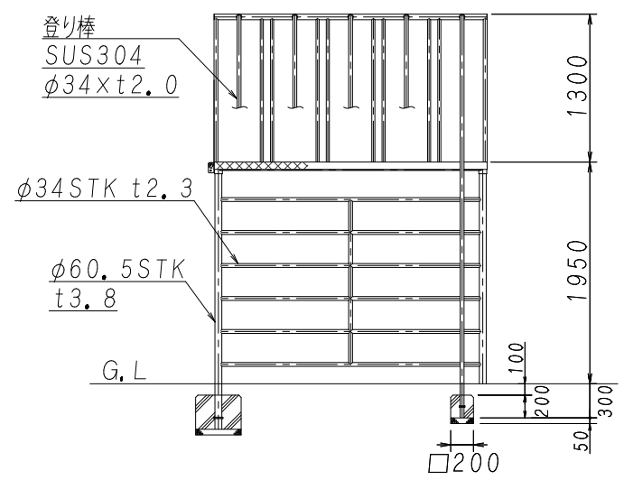
A ~ A 視図 S = 1 / 60
