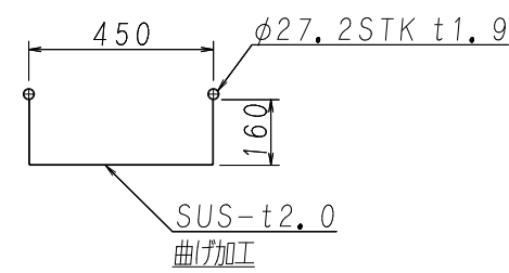
滑り面断面図 S = 1 / 20
