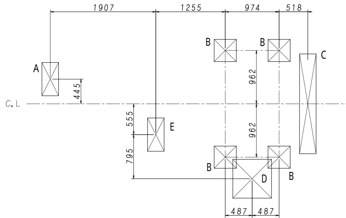
基礎平面図 S = 1/40
