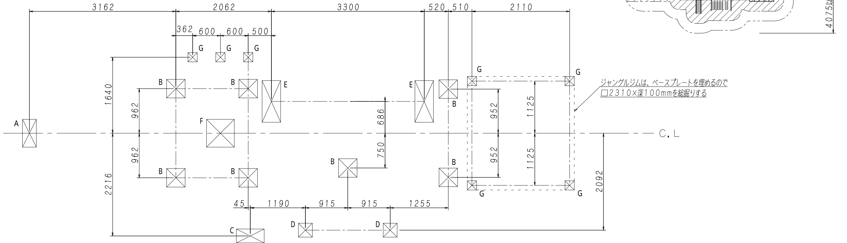
基礎平面図 S = 1 / 50
