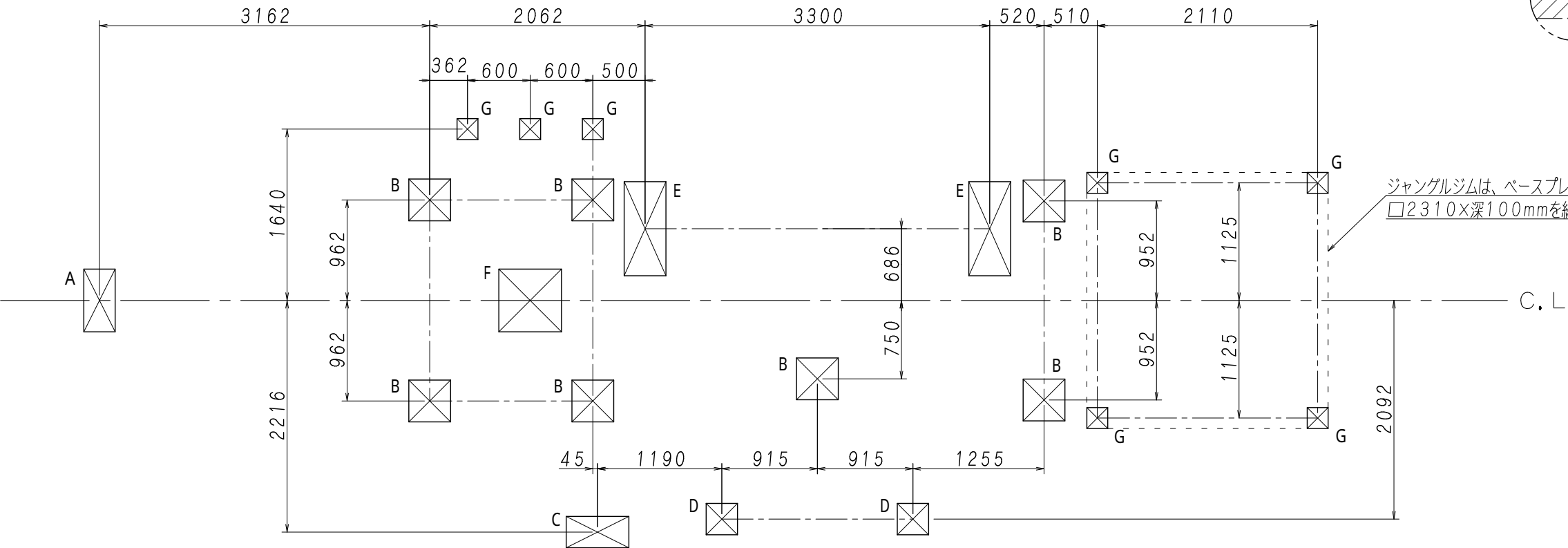
基礎平面図 S = 1 / 5 0
