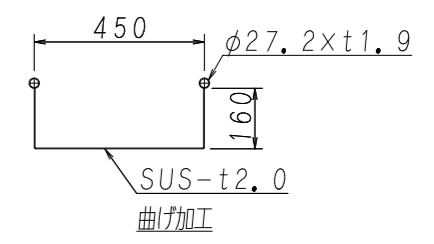
直線滑り面断面図 S = 1 / 20
