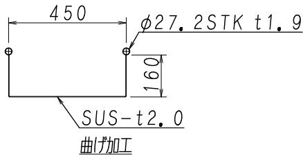
直線滑り面断面図 S=1/20
