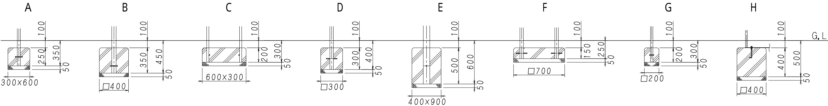
基礎断面図 S = 1/30
