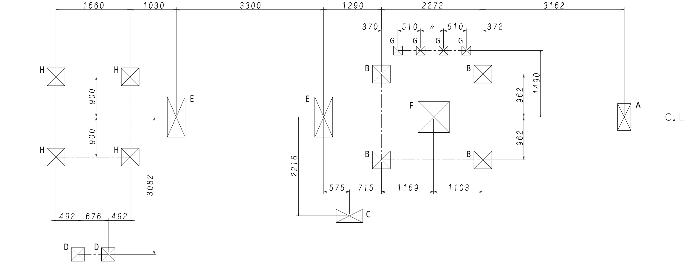
基礎平面図 S = 1/50
