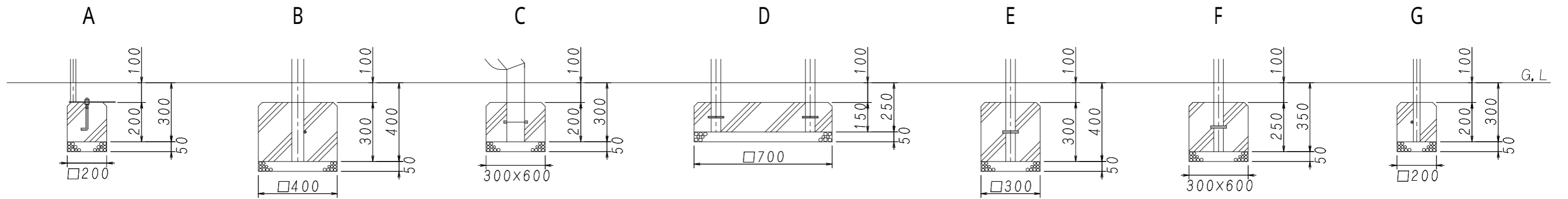
基礎断面図 S = 1/20
