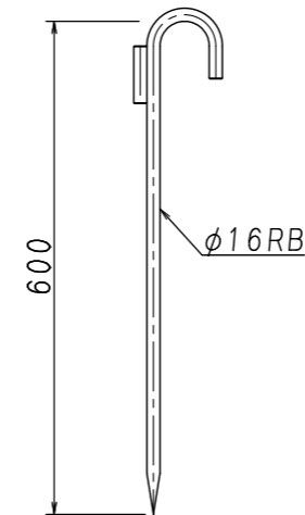
固定杭 S = 1/10 (半対につき4本)
