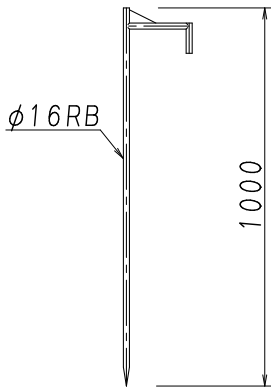
固定杭 × 3本
